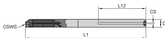
Barra de mandrinado de metal duro ajustable con conexión KM™.
